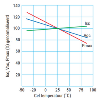
Temperatuursafhankelijkheid van Isc, Voc, Pmax
